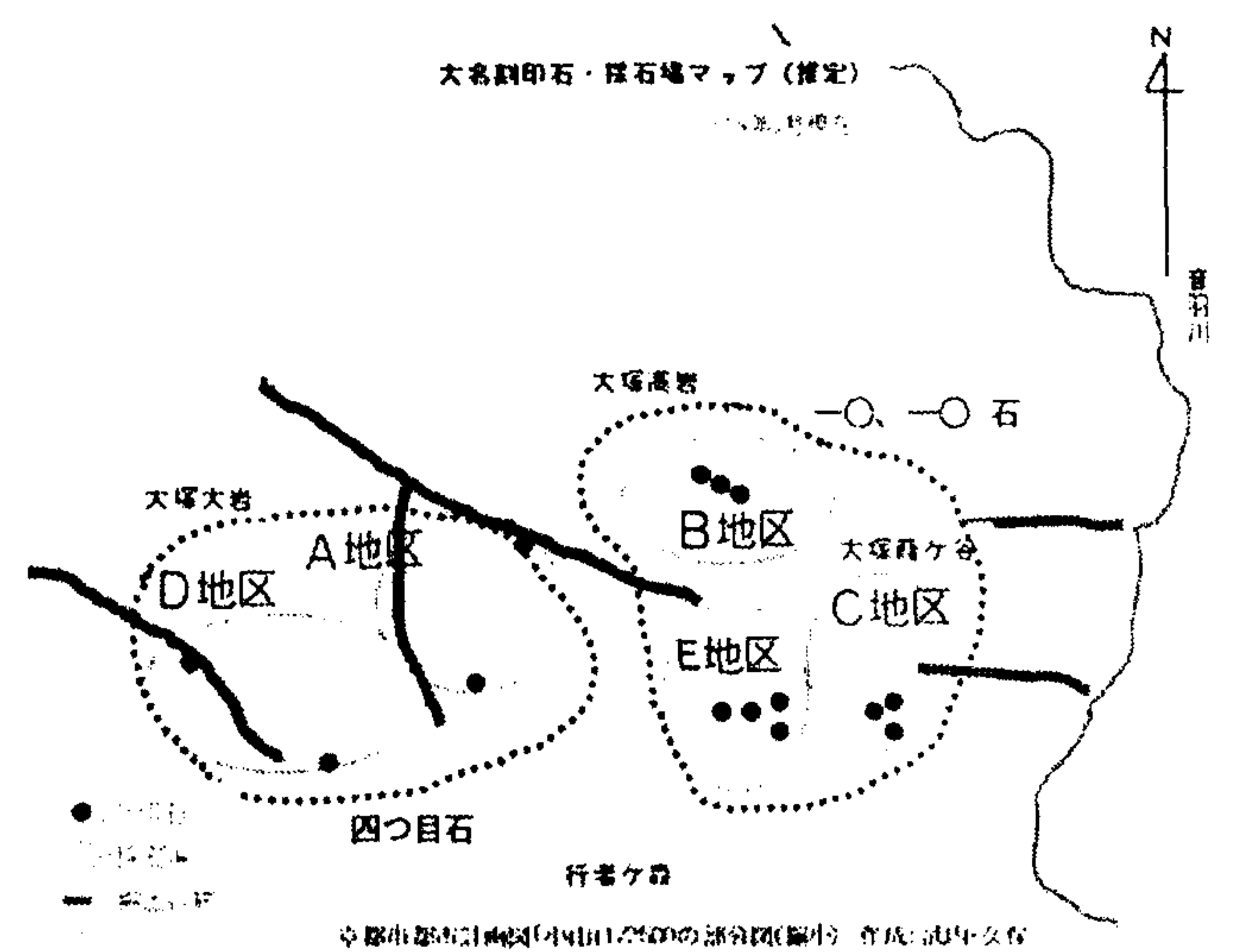
図2 山科区大塚山採石場跡地図
